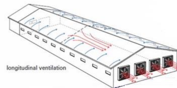
Schéma du système de ventilation
